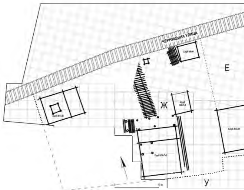
Рис. 4. Схема застройки усадьбы Ж периода V (1150–1190-е гг.)
