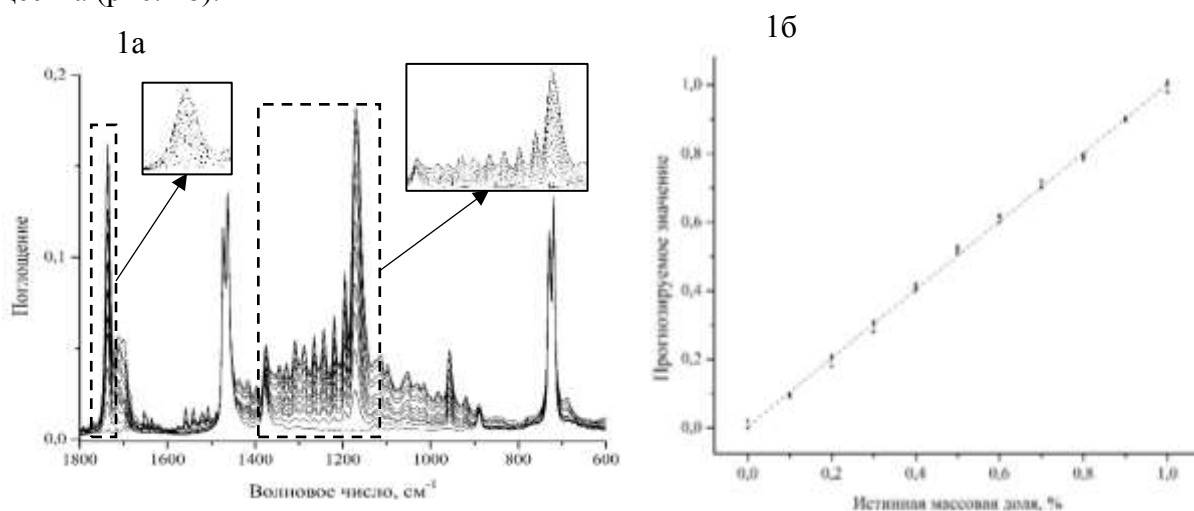
Рисунок 1 – ИК-Фурье спектр воска, парафина и смеси с содержанием парафина от 5 до 95 масс. % (1а). Калибровочный график значения доли парафина в составе по сравнению с прогнозируемым значением (1б)
